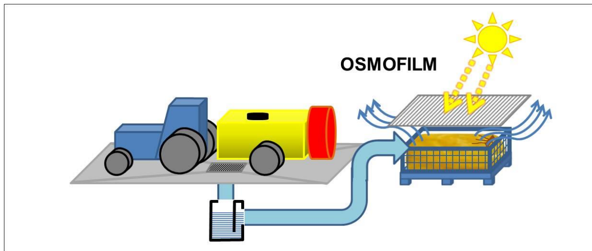
Rys. 52. Stanowisko OSMOFILM
